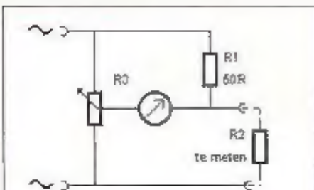
Figuur 1. Voor het bepalen van de grootte van R_2 draai je net zolang aan potmeter R_3 totdat de meter niet meer uitslaat; de brug is dan in evenwicht. De weerstandsverhouding in R_3 is dan gelijk aan die tussen R_1 en R_2 waarbij R_1 een bekende waarde heeft. Uit de stand van de loper van R_3 volgt de waarde van de onbekende R_2 .
